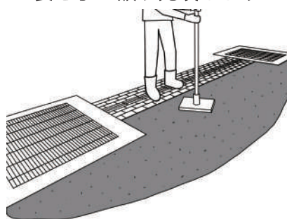
5. 転圧 タンパーや足で転圧します
